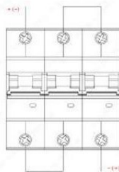
3P外形
