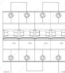
4P外形
